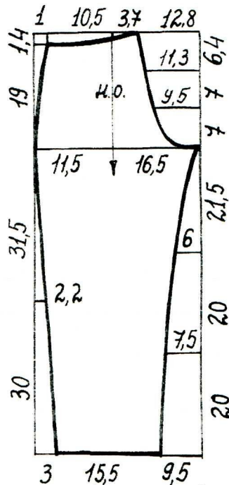
Задняя половинка брюк
